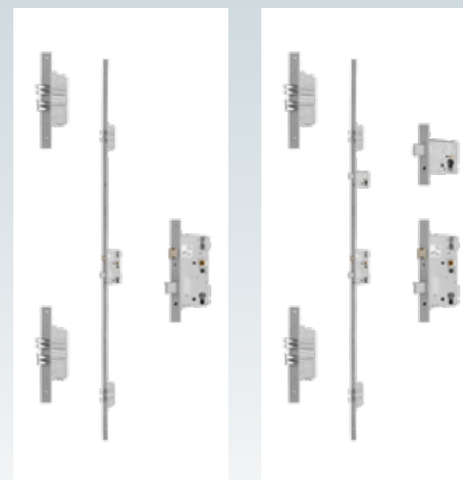
Zamek listwowy ROTO QB (3 zamki)
